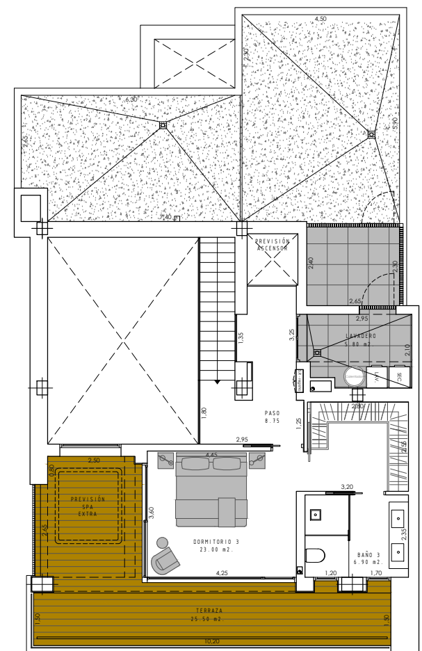
PLANTA ALTA
