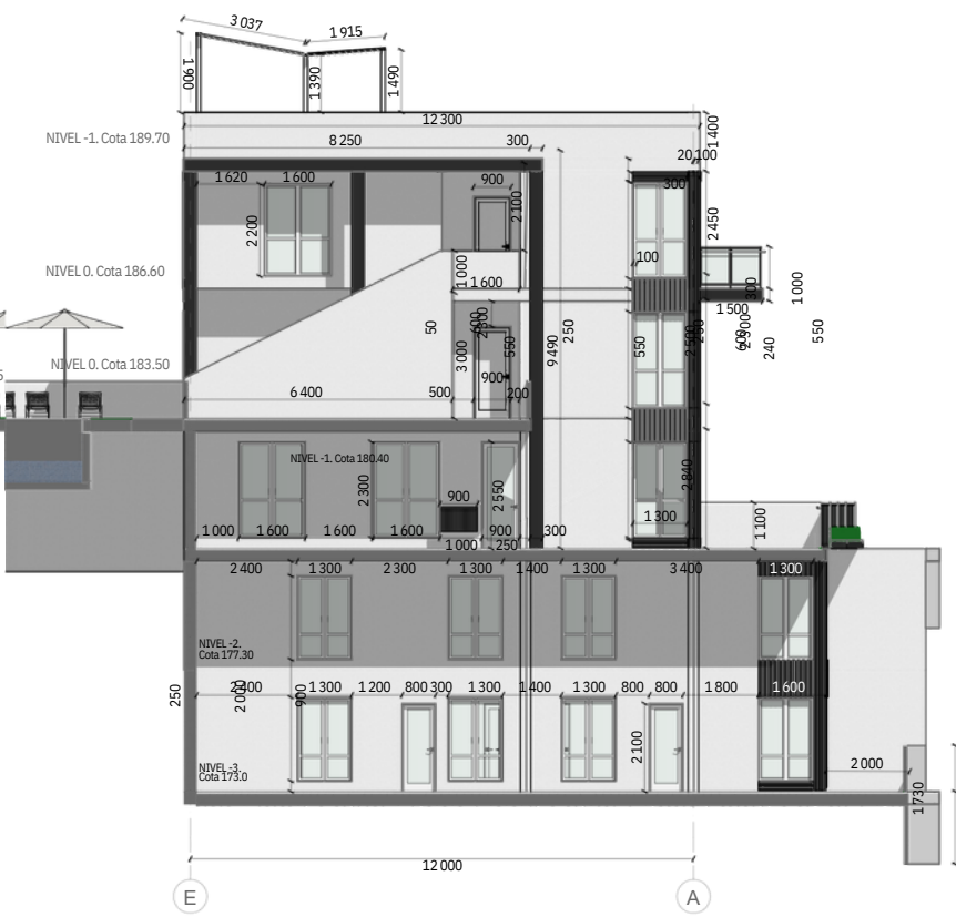
ALZADO IZQUIERDO
