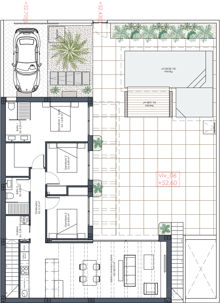
PLANTA BAJA
