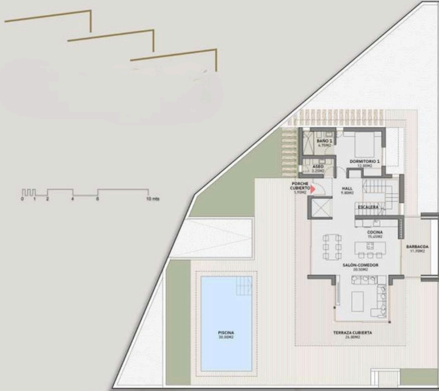
PLANTA BAJA
