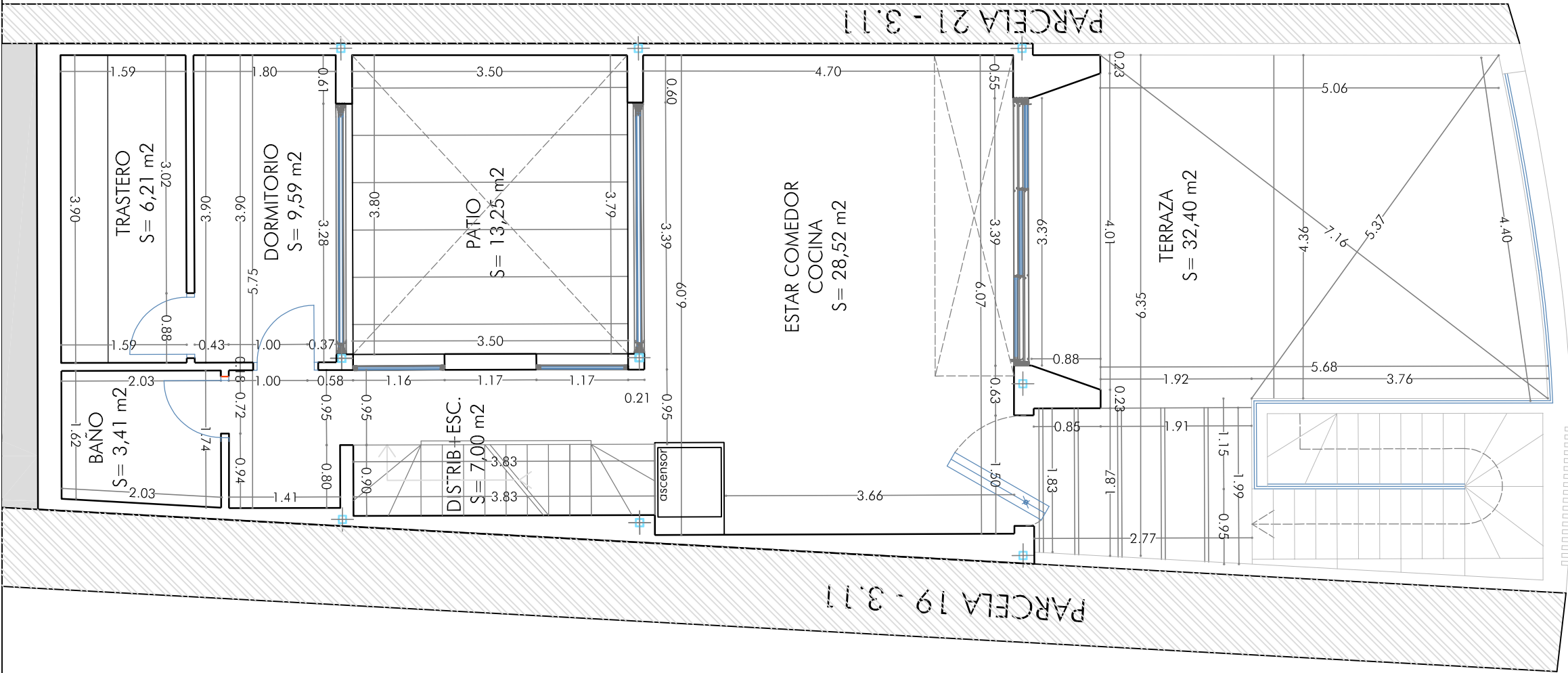
PLANTA BAJA: COTAS Y SUPERFICIES
