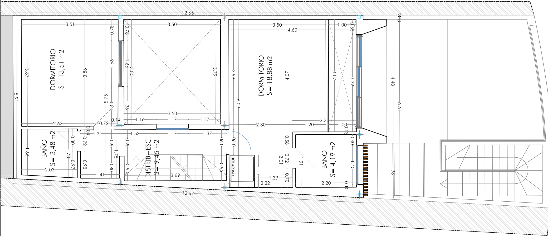
PLANTA PRIMERA: COTAS Y SUPERFICIES
