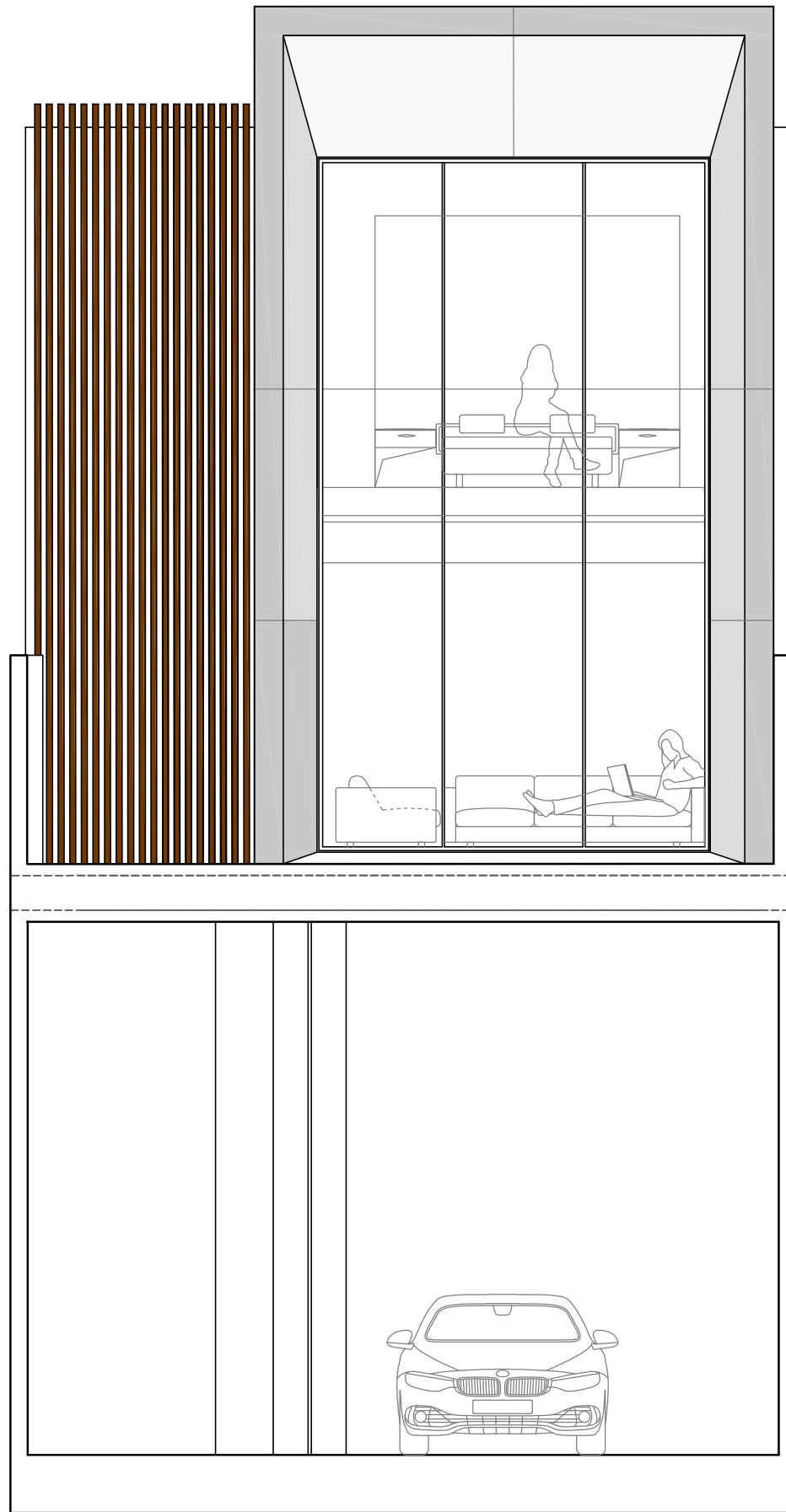
PARCELA 20 - 3.11 -SECCIÓN ALZADO SUR
