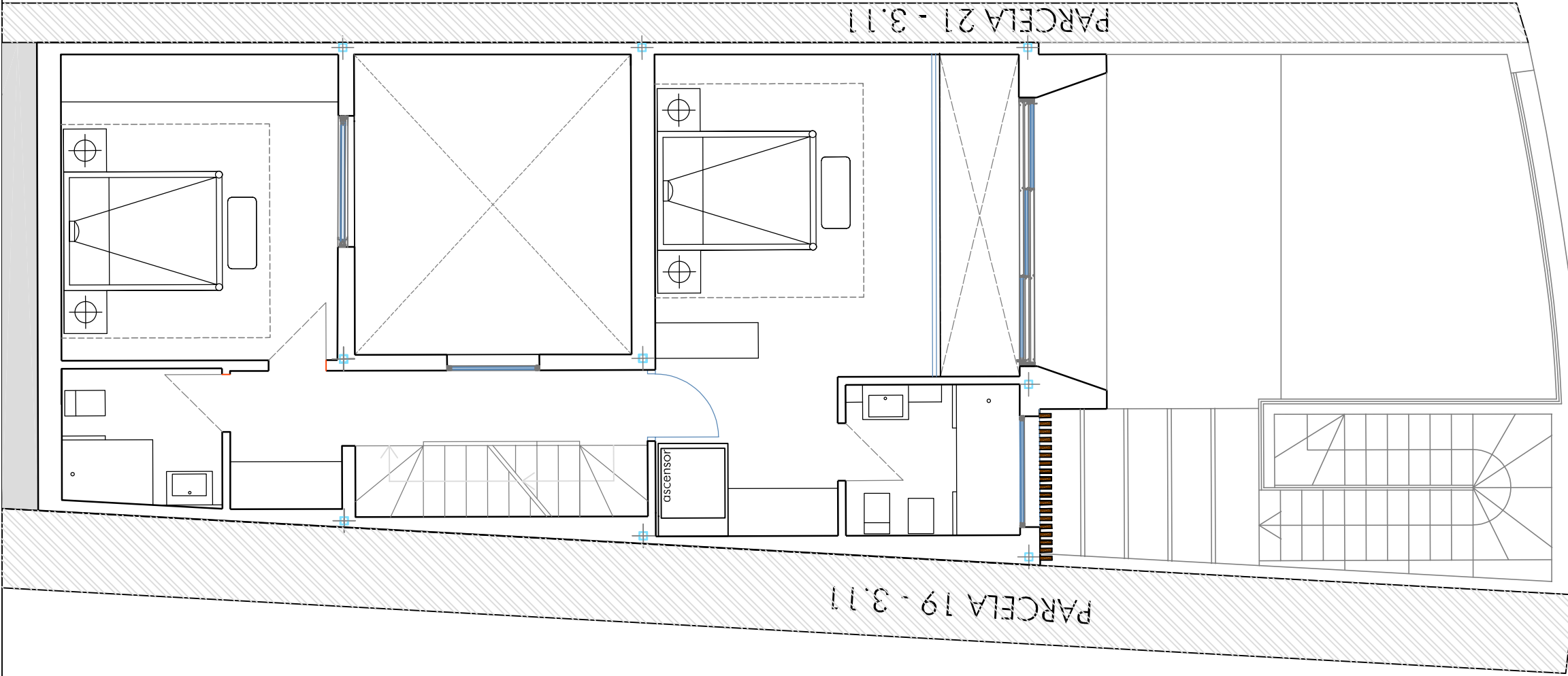
PLANTA PRIMERA: DISTRIBUCIÓN Y USOS
