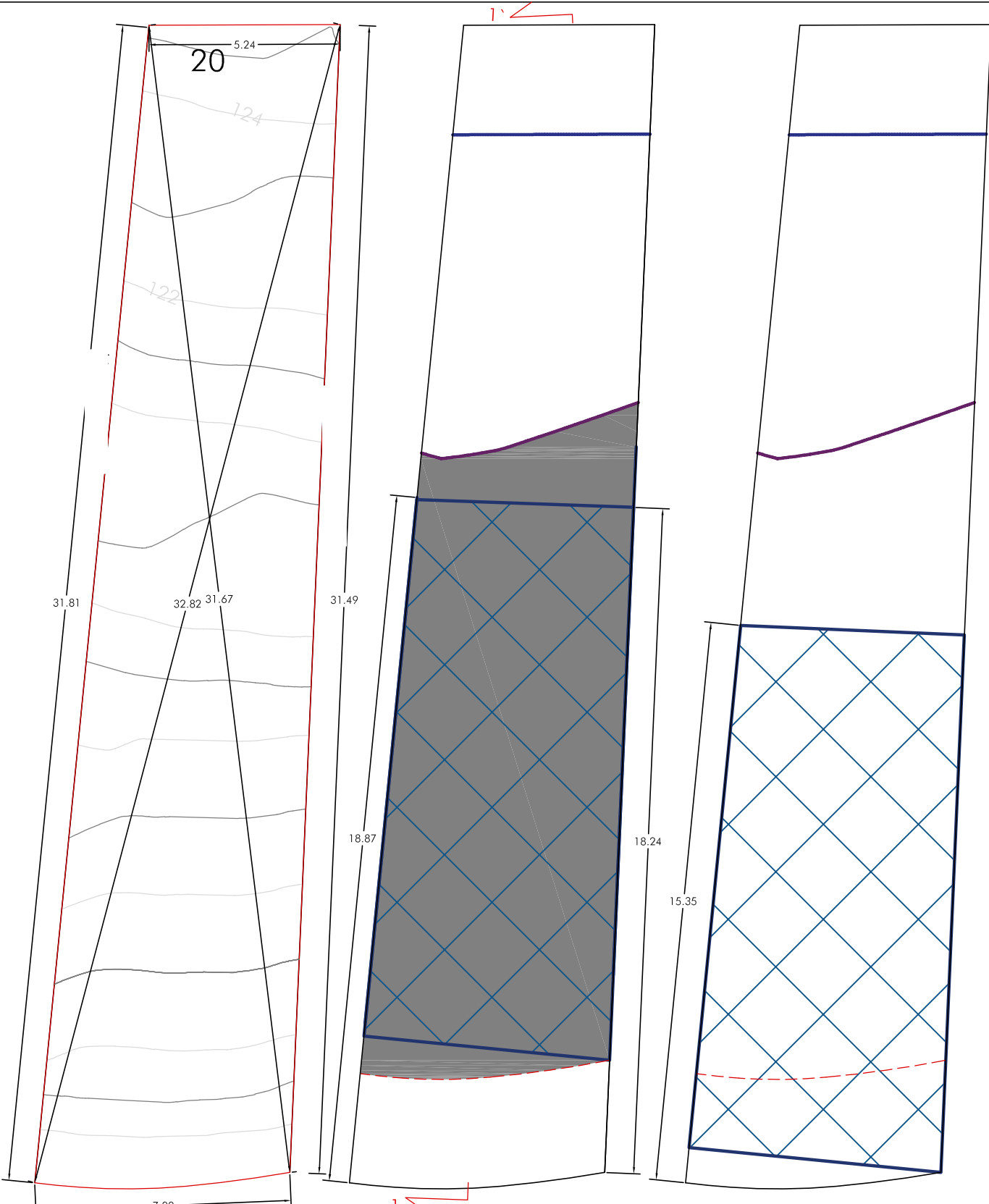
PARCELA 20 - 3.11 - TOPOGRÁFICO ACTUAL GEOMETRÍA Y SUPERFICIES PARCELA 20 - 3.11 - ALINEACIONES PARCELA 20 - 3.11 - ALINEACIONES PLANTA GARAJE
