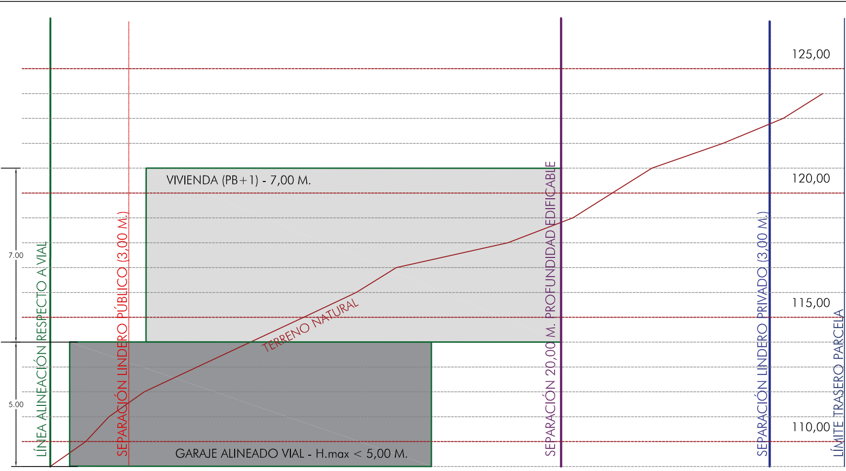
PARCELA 20 - 3.11 - SECCIÓN 1-1'
