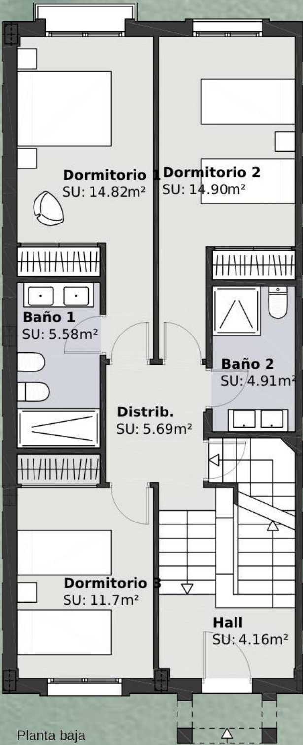
Planta baja
