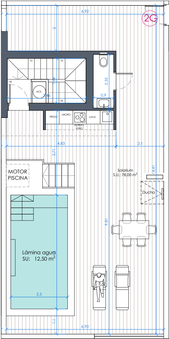
Planta Solarium
