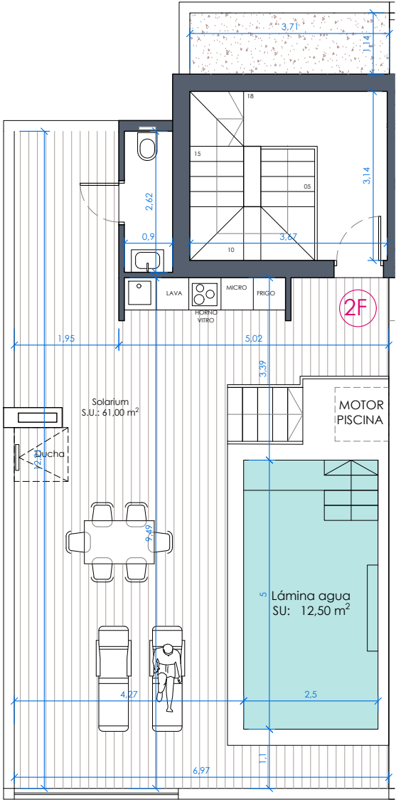
Planta Solarium
