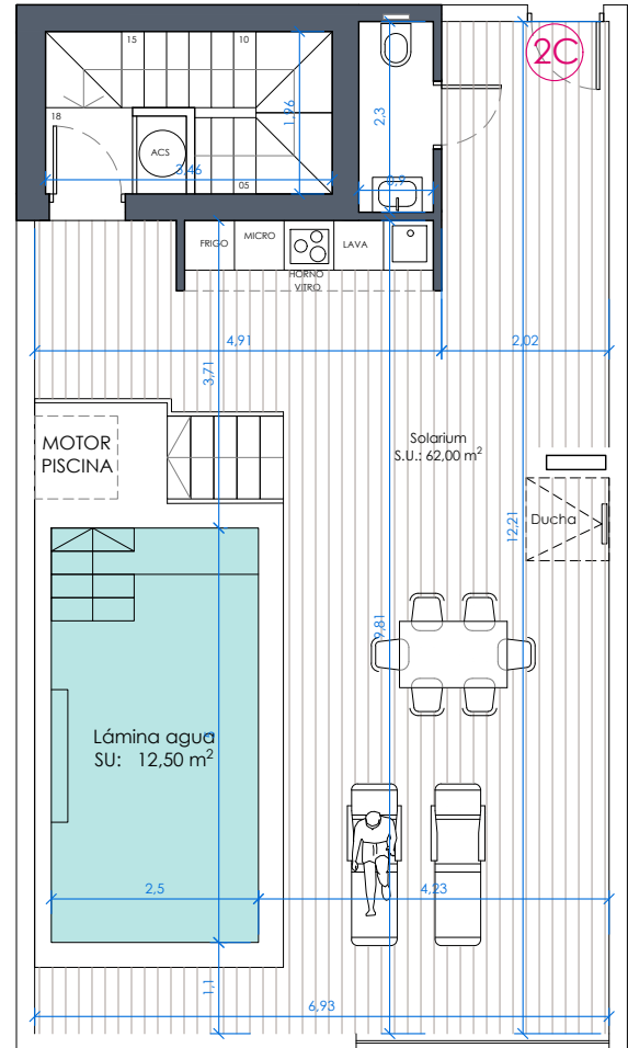
Planta Solarium
