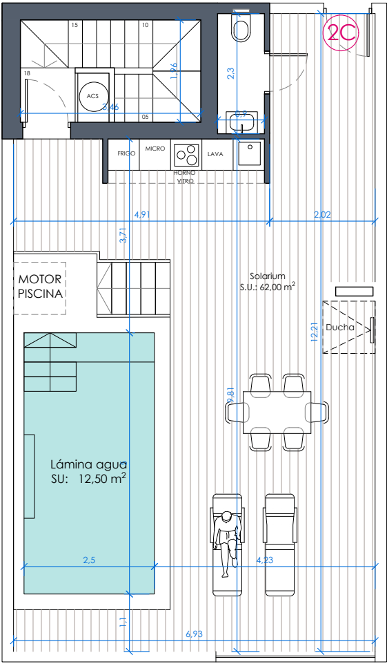
Planta Solarium
