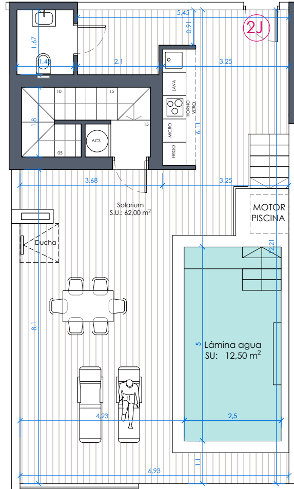
Planta Solarium
