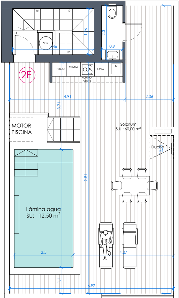
Planta Solarium
