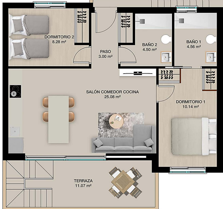
PLANTA PRIMERA FIRST FLOOR
