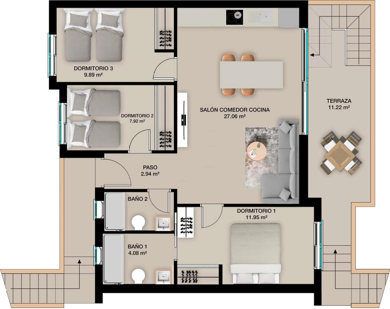
PLANTA PRIMERA
