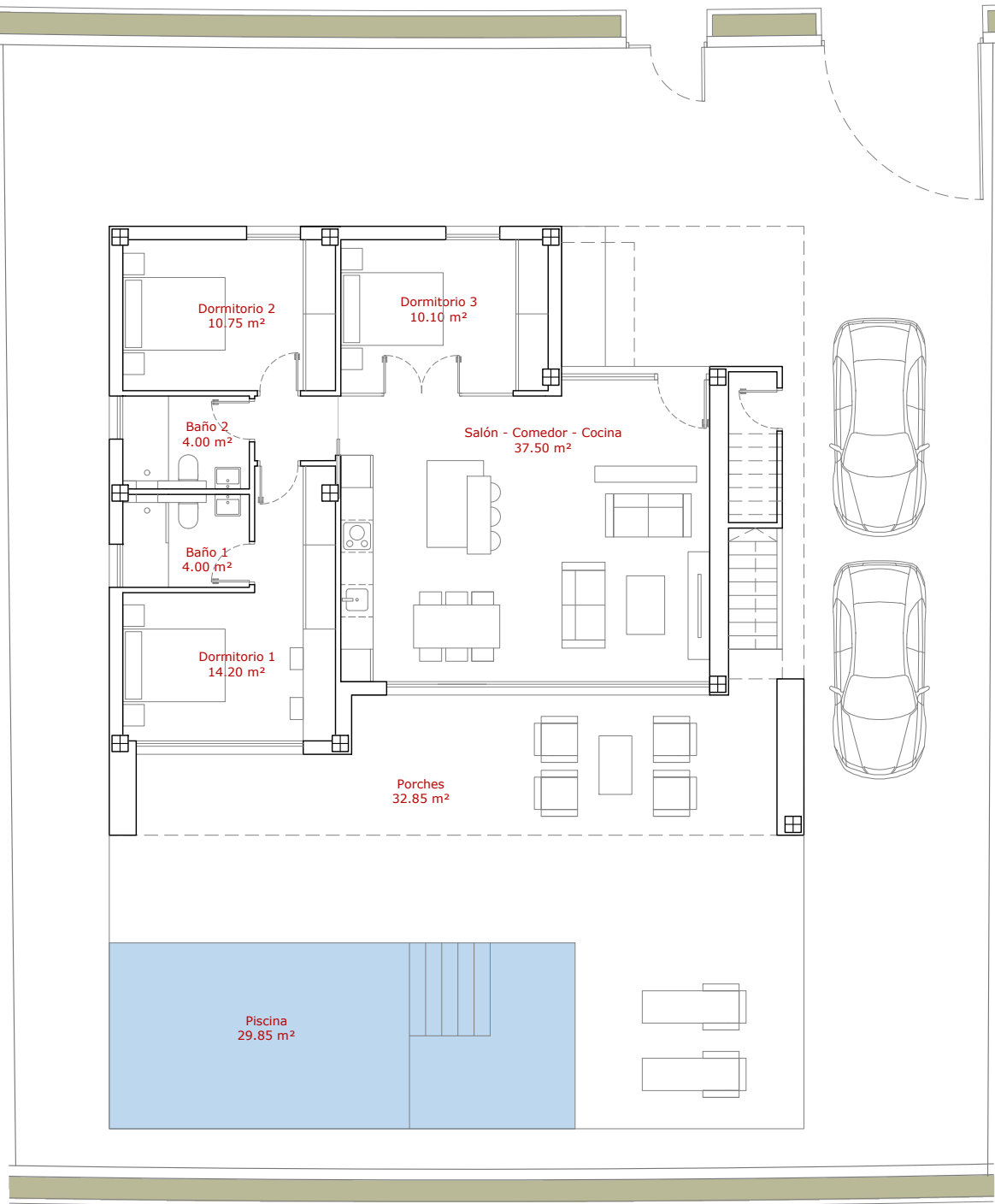
Planta Baja
