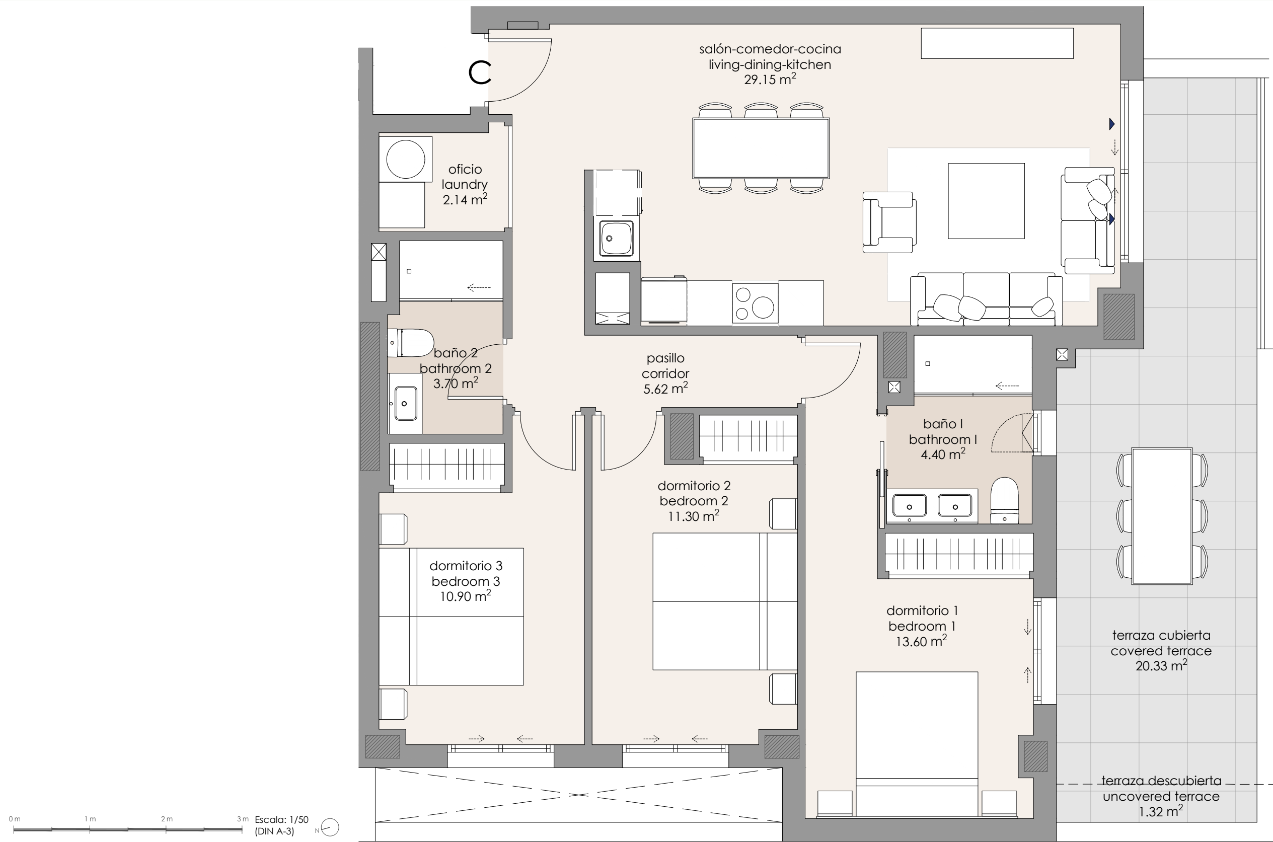
Plano de Vivienda Edificio B - Pl. 1ª - C Flat Building B - First floor - C Floorplan 3 Dormitorios + terraza 3 Bedrooms + terrace
