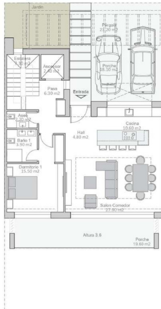
PLANTA/PRIMERERA First floor
