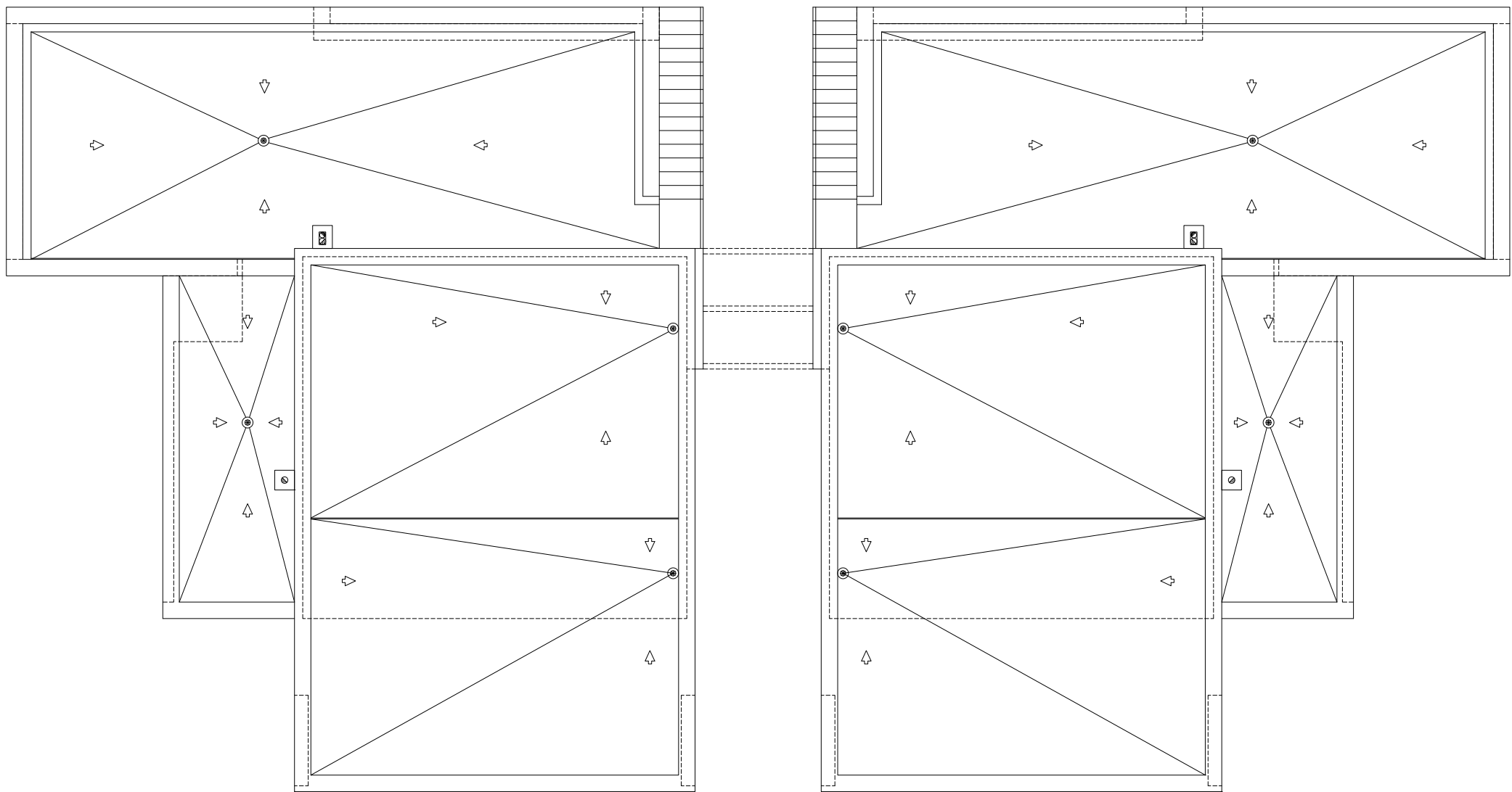
PLANTA CUBIERTA
