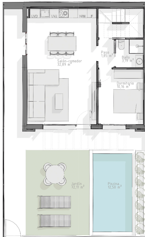
8.Viv. Unifamiliar. Planta baja
