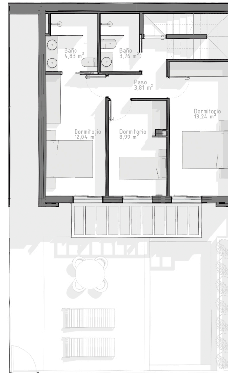
8.Viv. Unifamiliar. Planta 1ª
