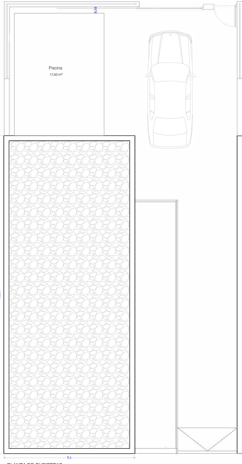
PLANTA DE CUBIERTAS
