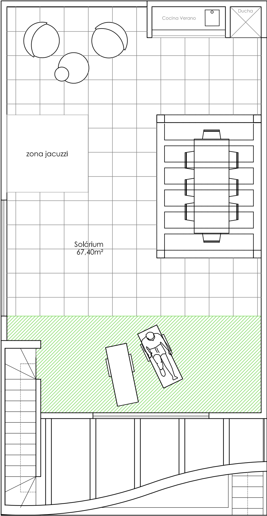
Planta Solárium
