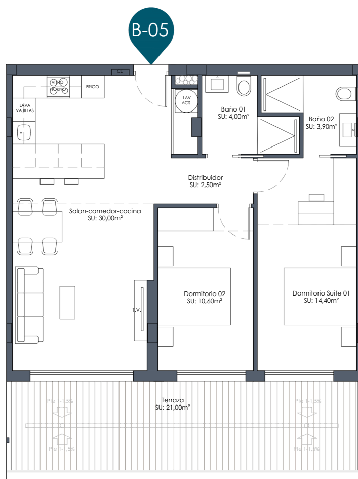
PLANTA PRIMERA
