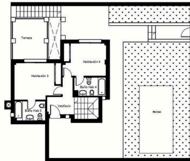
PLANTA PRIMERA
