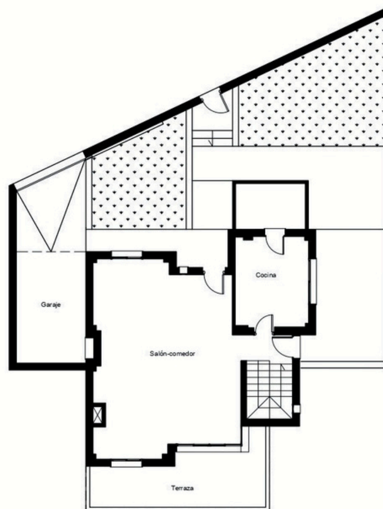
PLANTA BAJA
