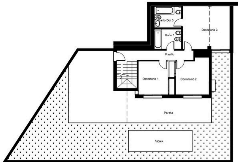
PLANTA SEMISÓTANO
