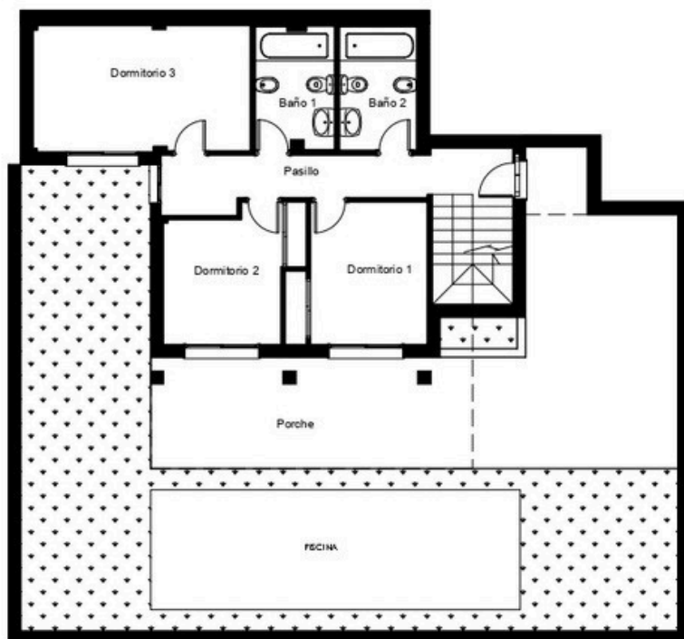
PLANTA SEMISÓTANO
