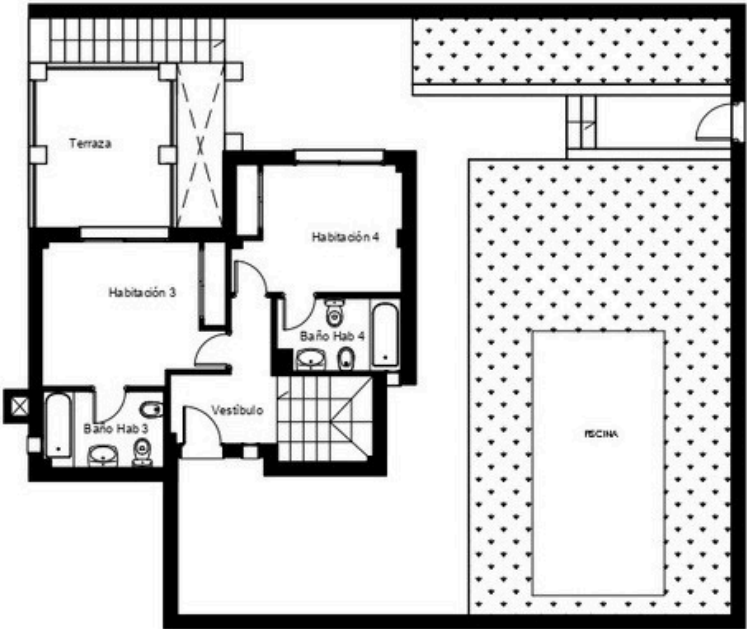
PLANTA PRIMERA
