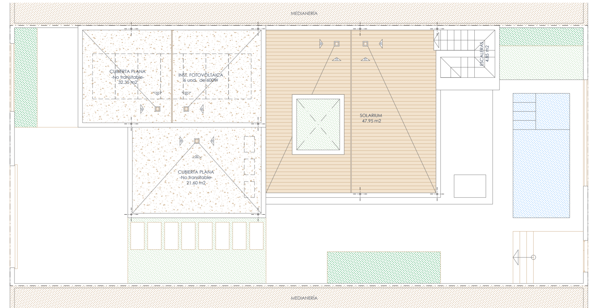
Planta Cubiertas
