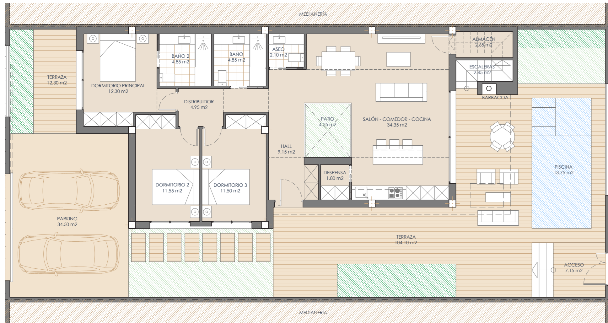
Planta Baja
