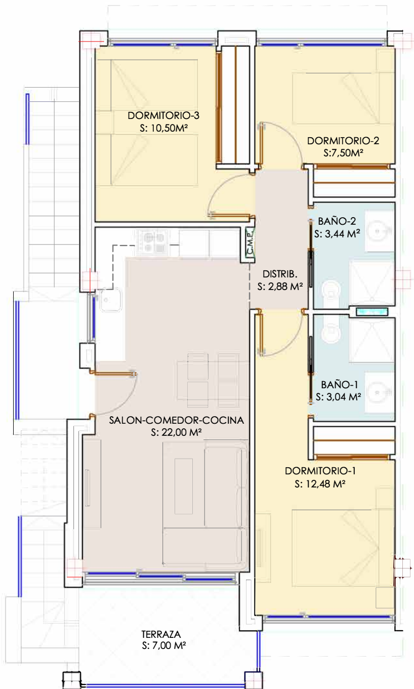
PLANTA PRIMERA
