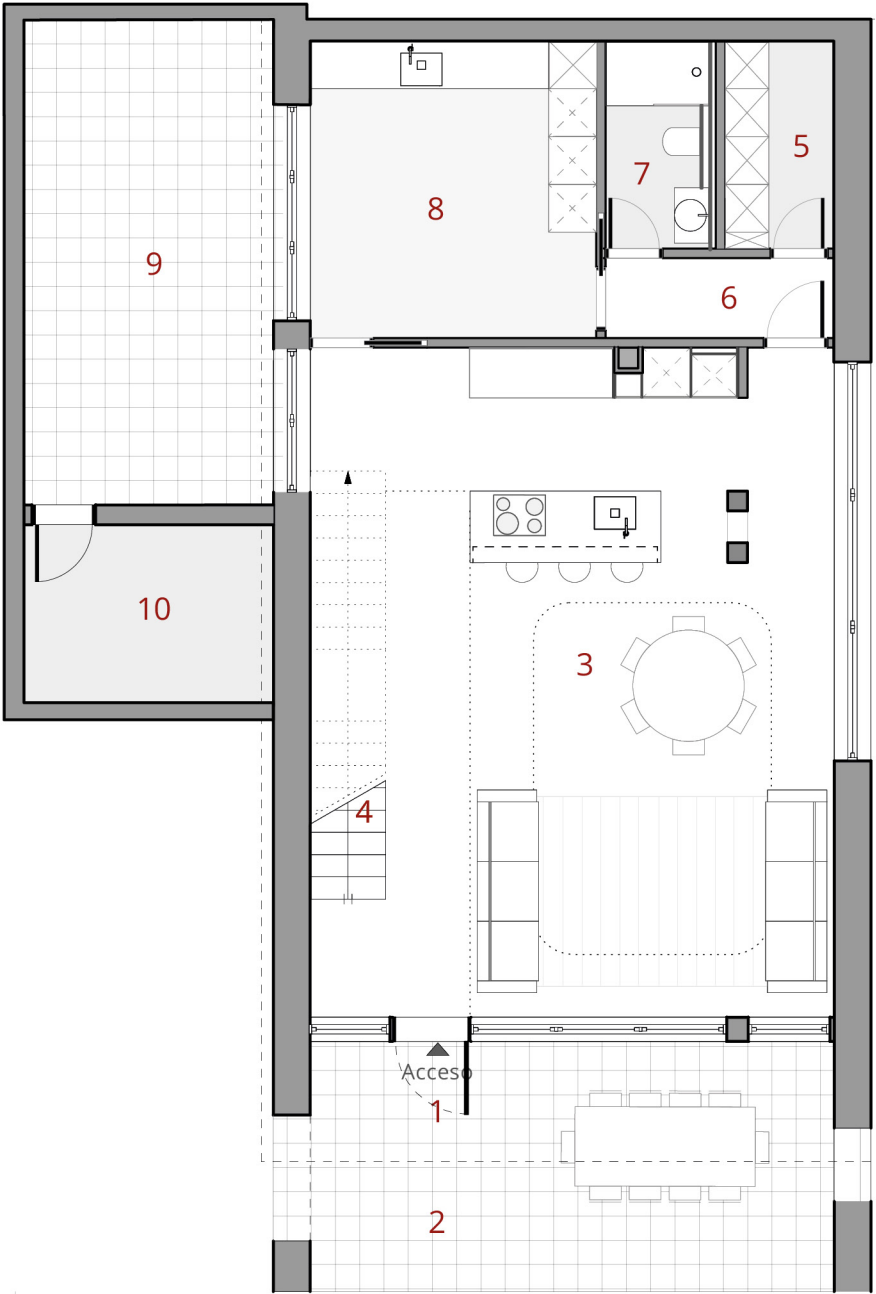
SUPERFICIE CONSTRUIDA VIVIENDA Planta Baja 108,10 m² (NO SE INCLUYEN TERRAZAS)
