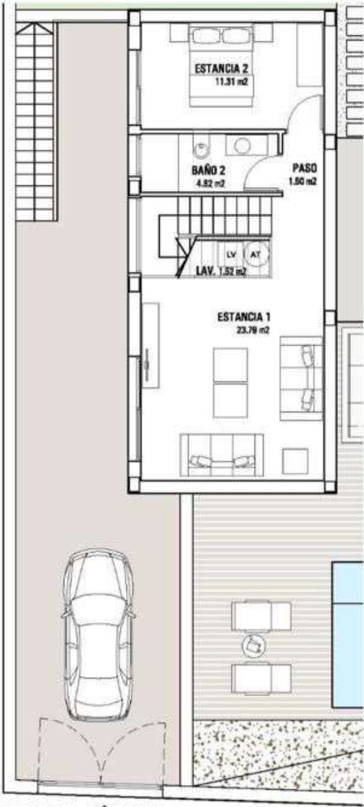
PLANTA SÓTANO
