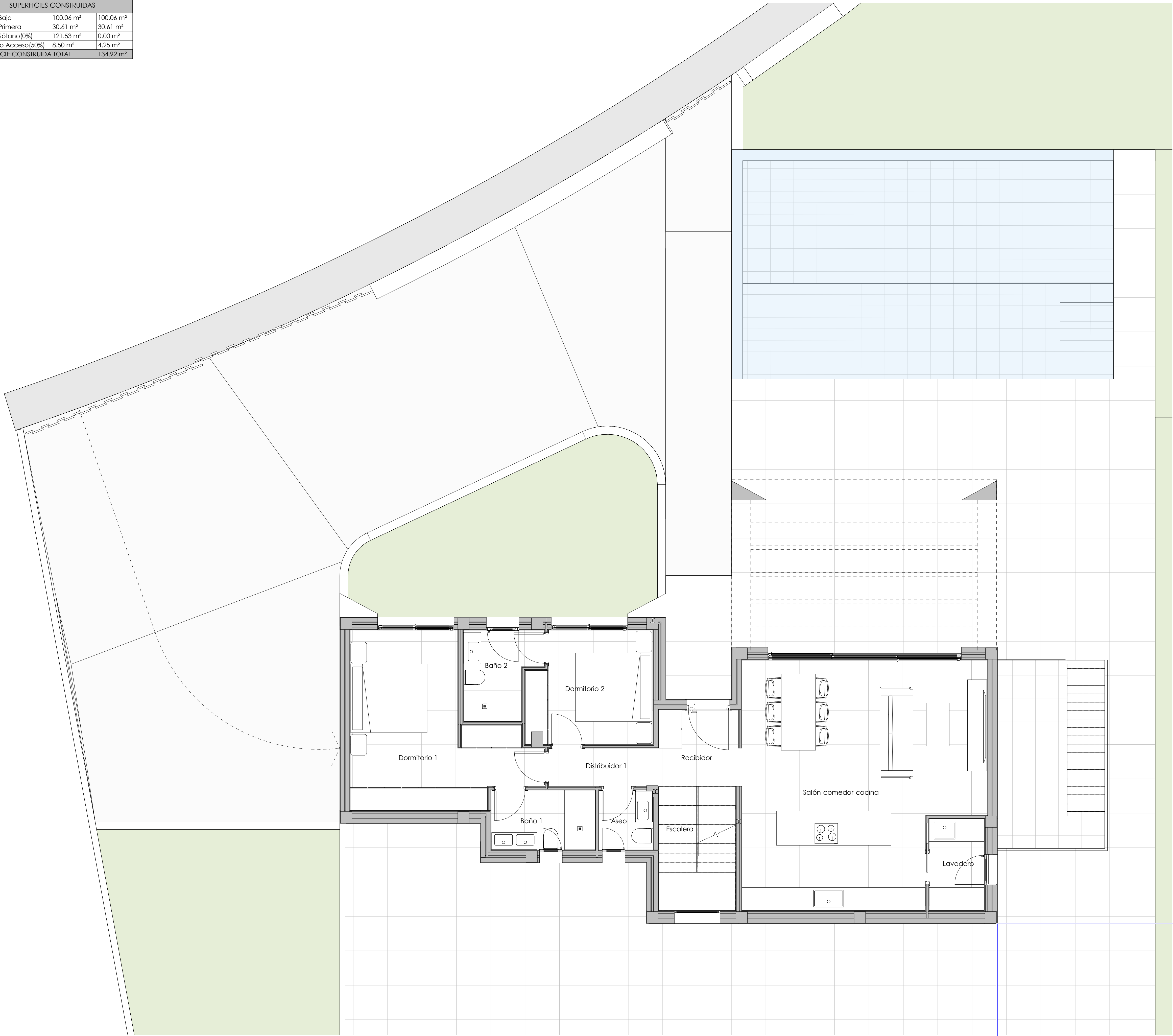
PLANTA BAJA
