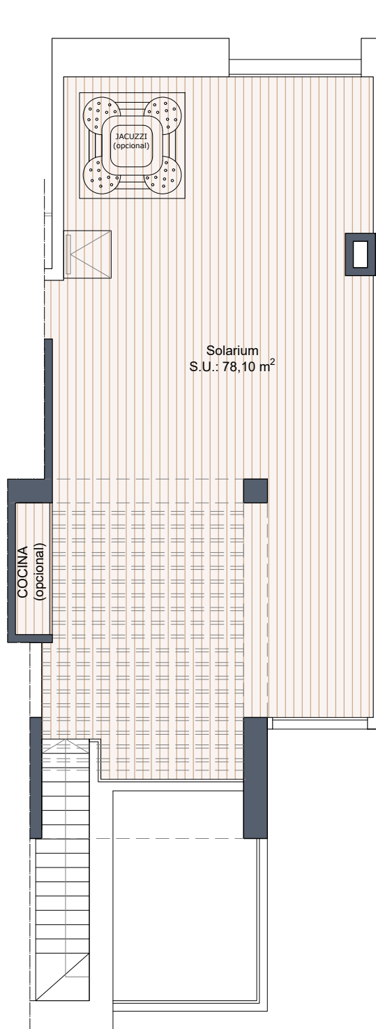
Planta solarium
