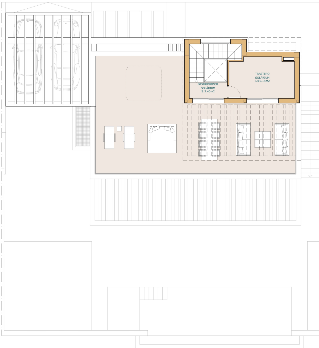
PLANTA SOLÁRIUM
