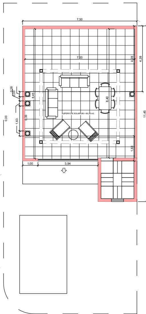
PLANTA SOLARIUM
