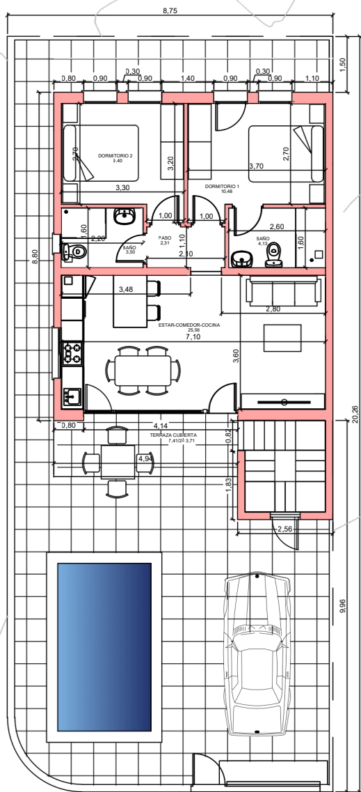
PLANTA BAJA
