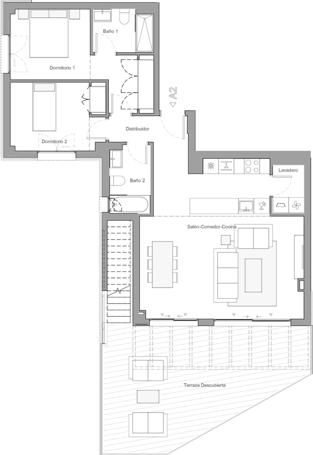
PORTAL 3 - PLANTA 2 - VIVIENDA A2
