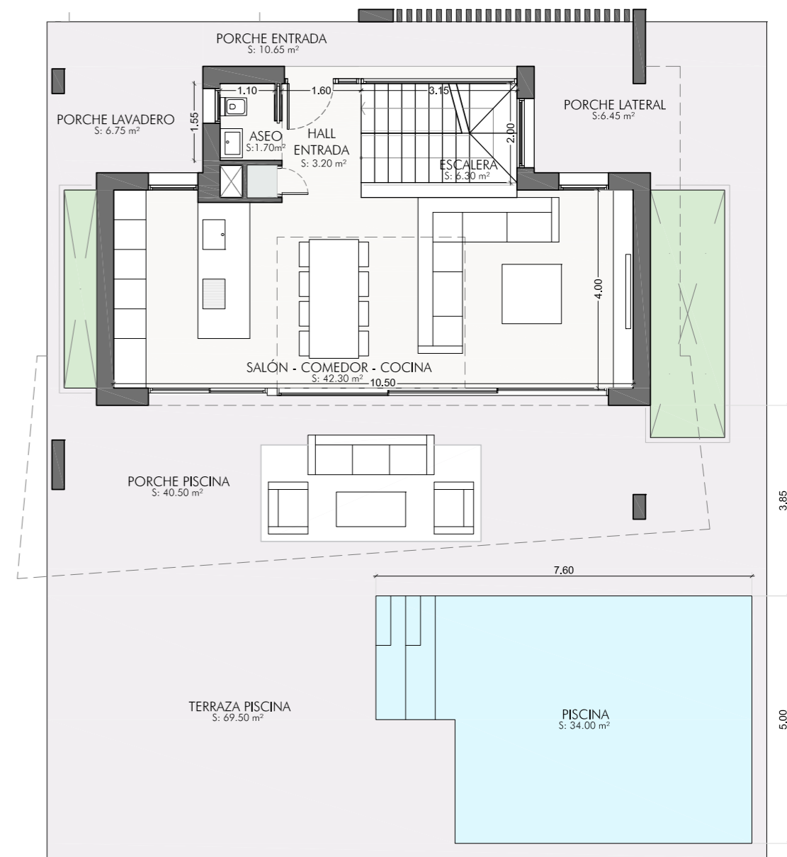
Planta Baja
