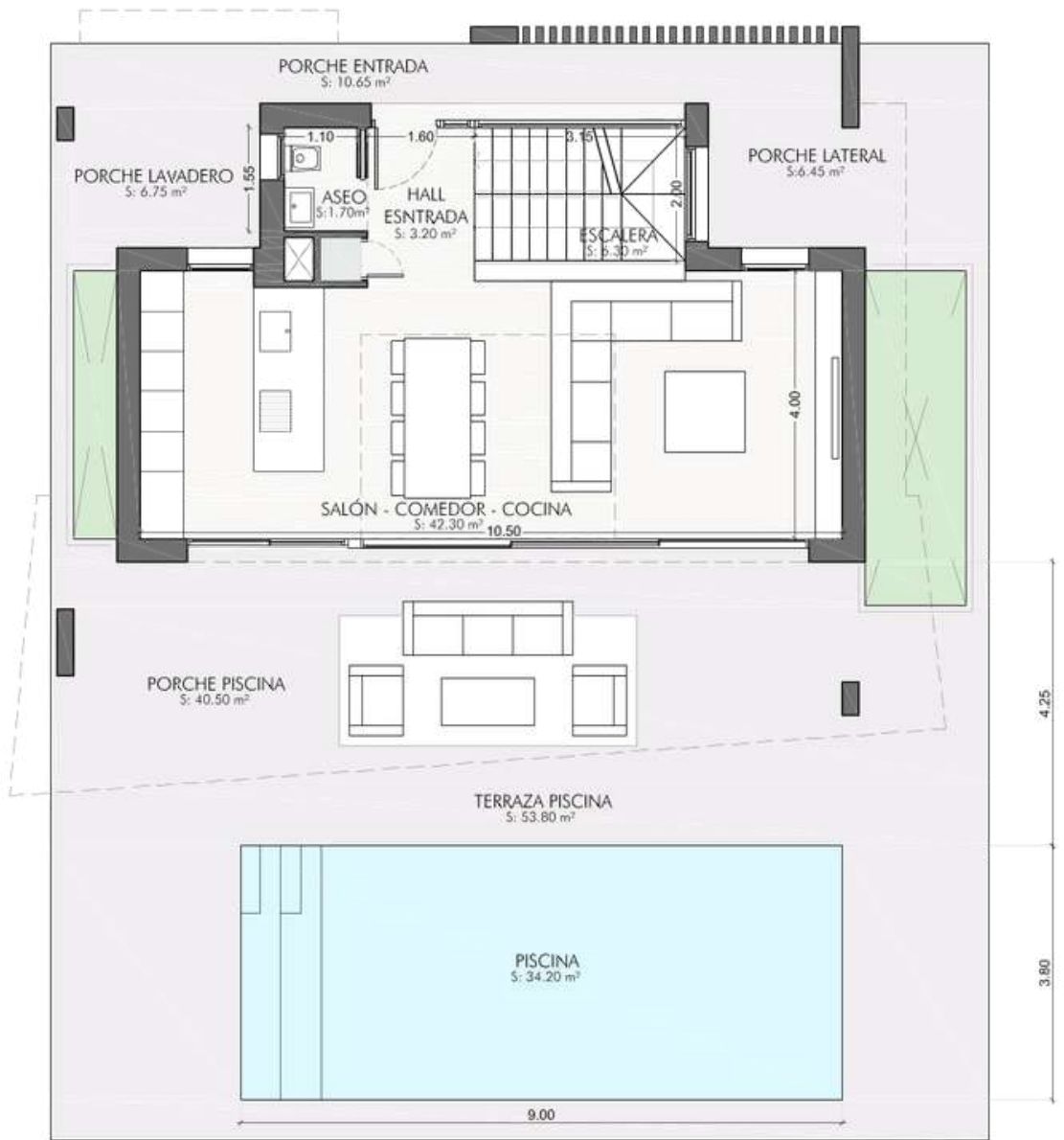
Planta Baja
