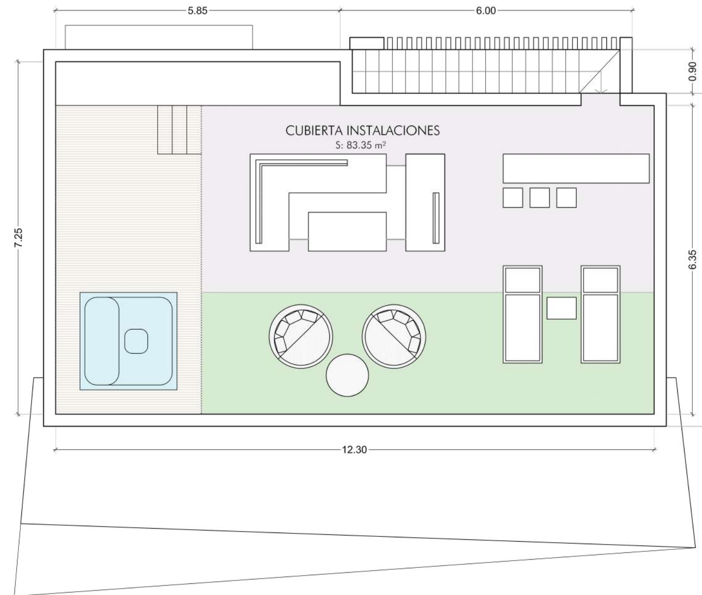
Planta Solarium
