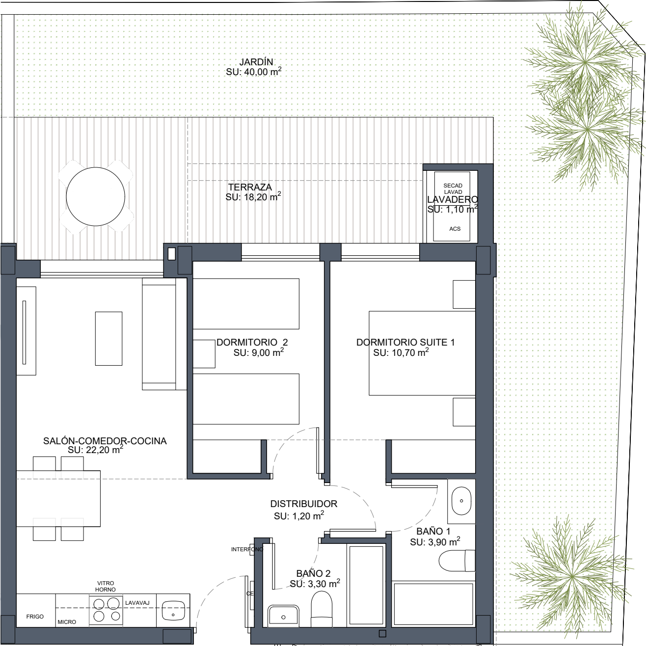
PLANTA BAJA
