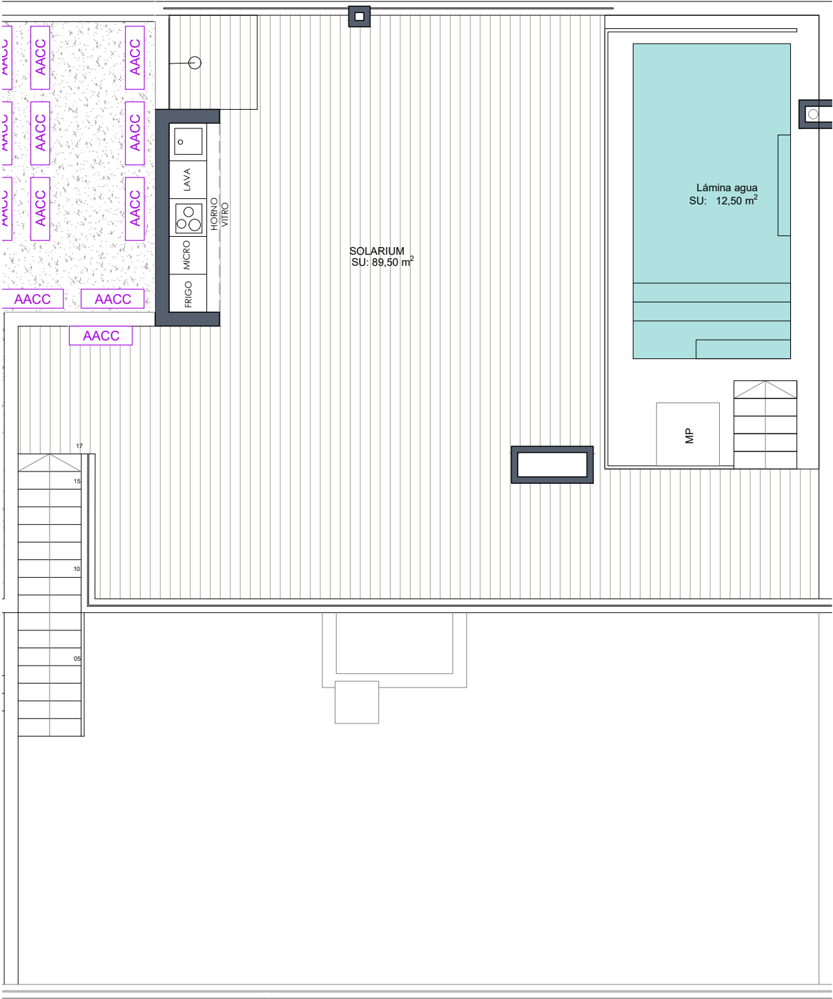
PLANTA SEGUNDA-SOLARIUM
