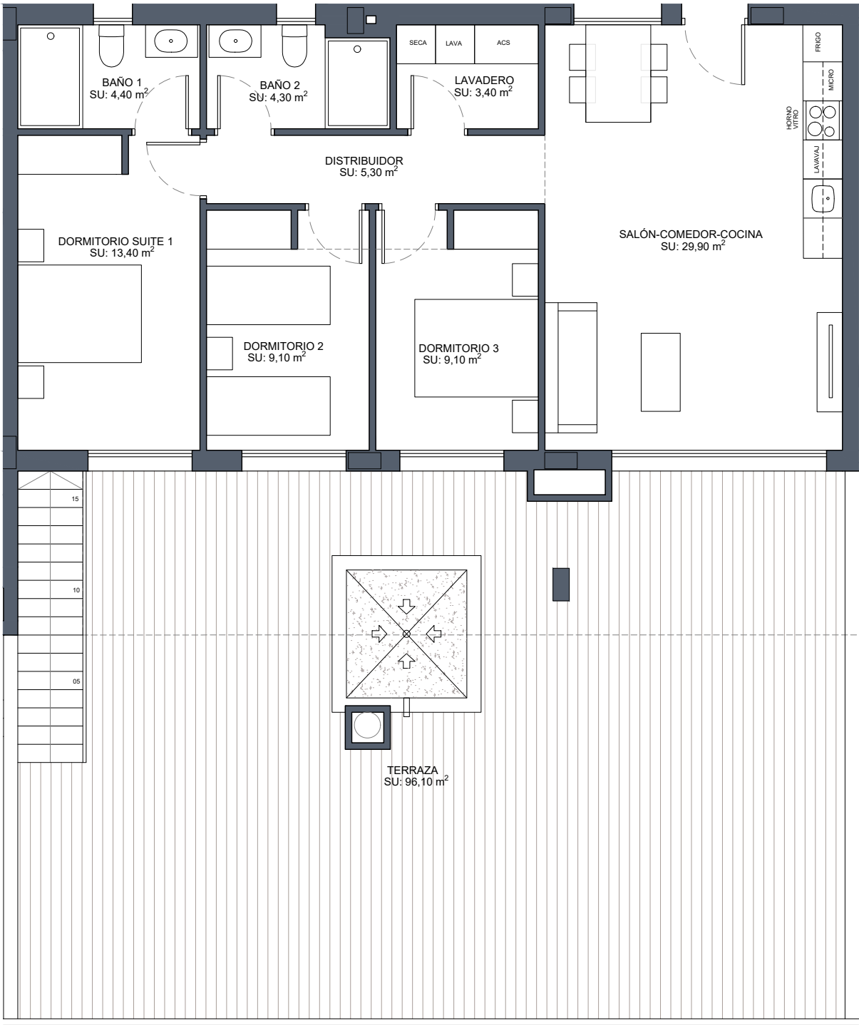
PLANTA SEGUNDA
